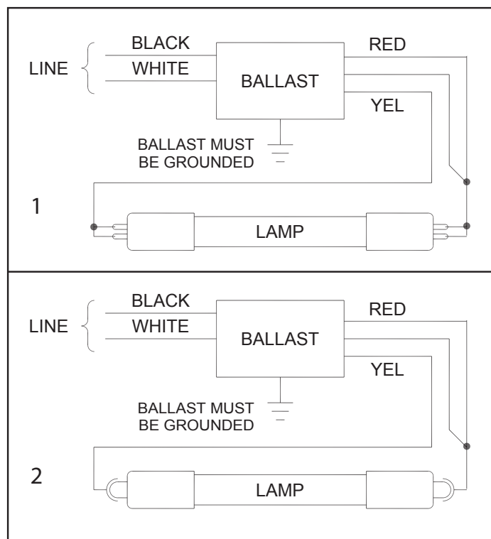
Wiring Diagrams
